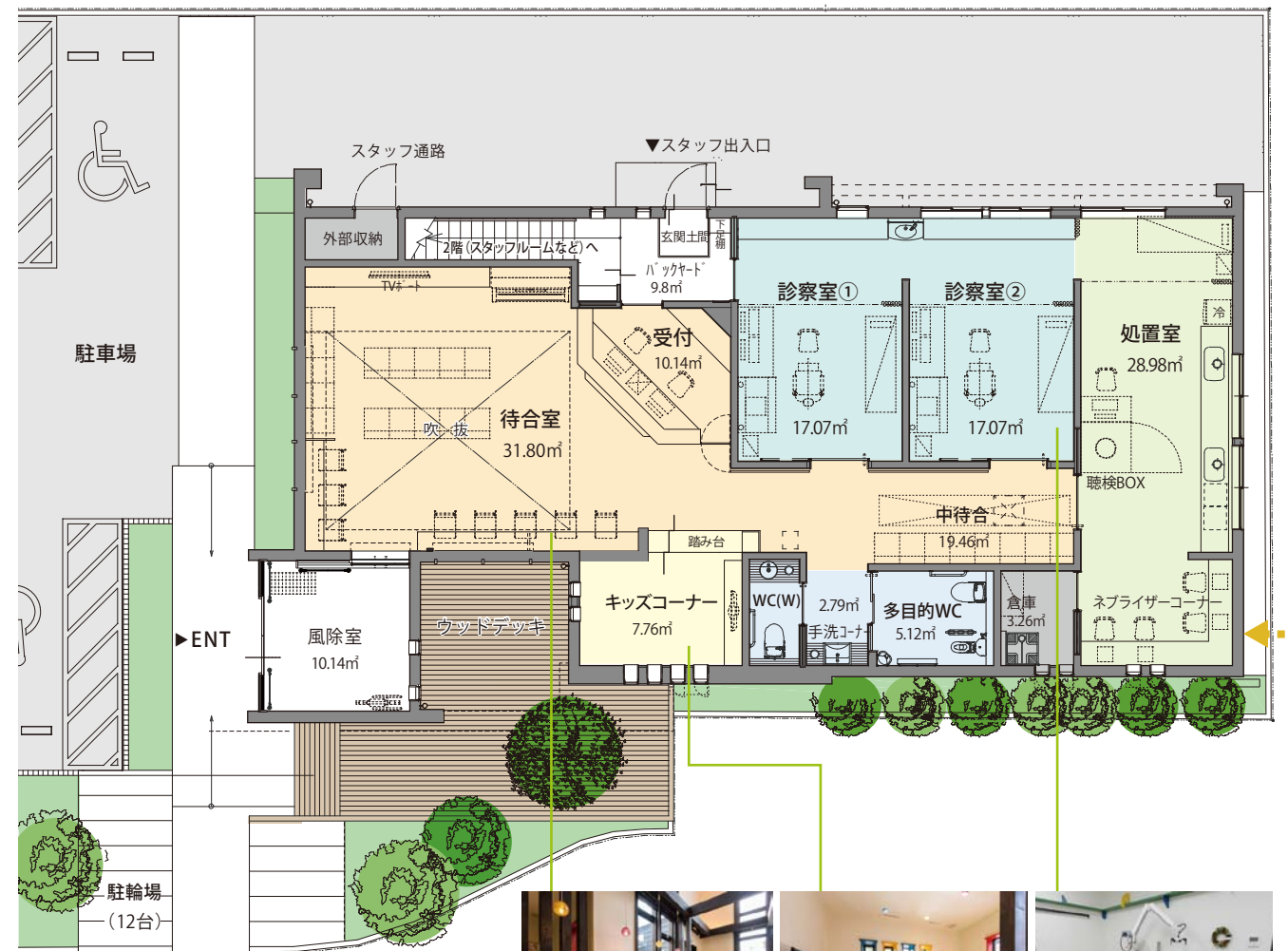
配置図
