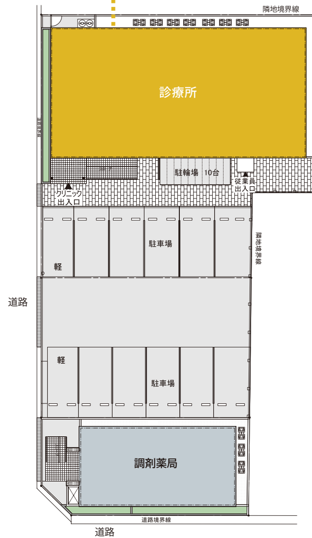
配置図
