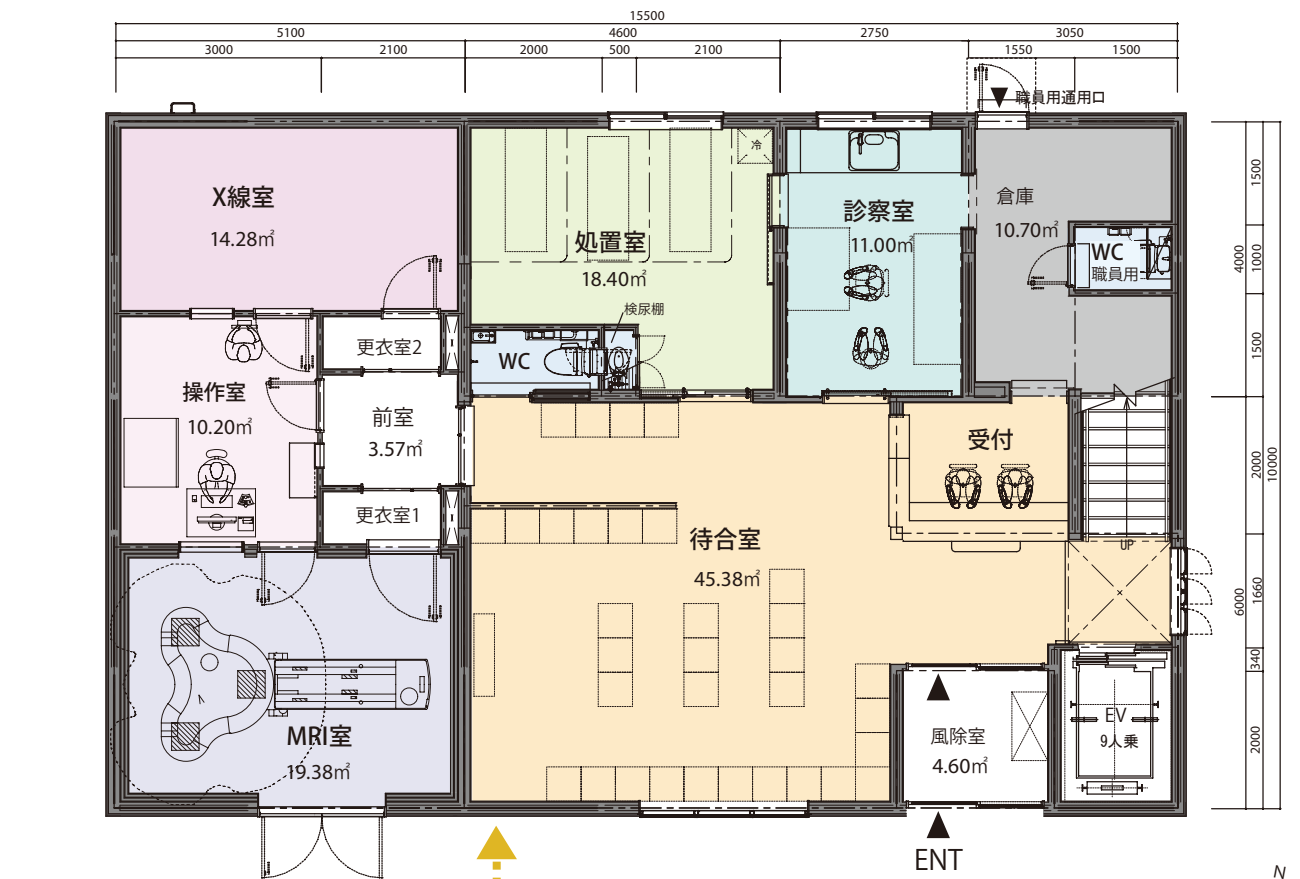
配置図
