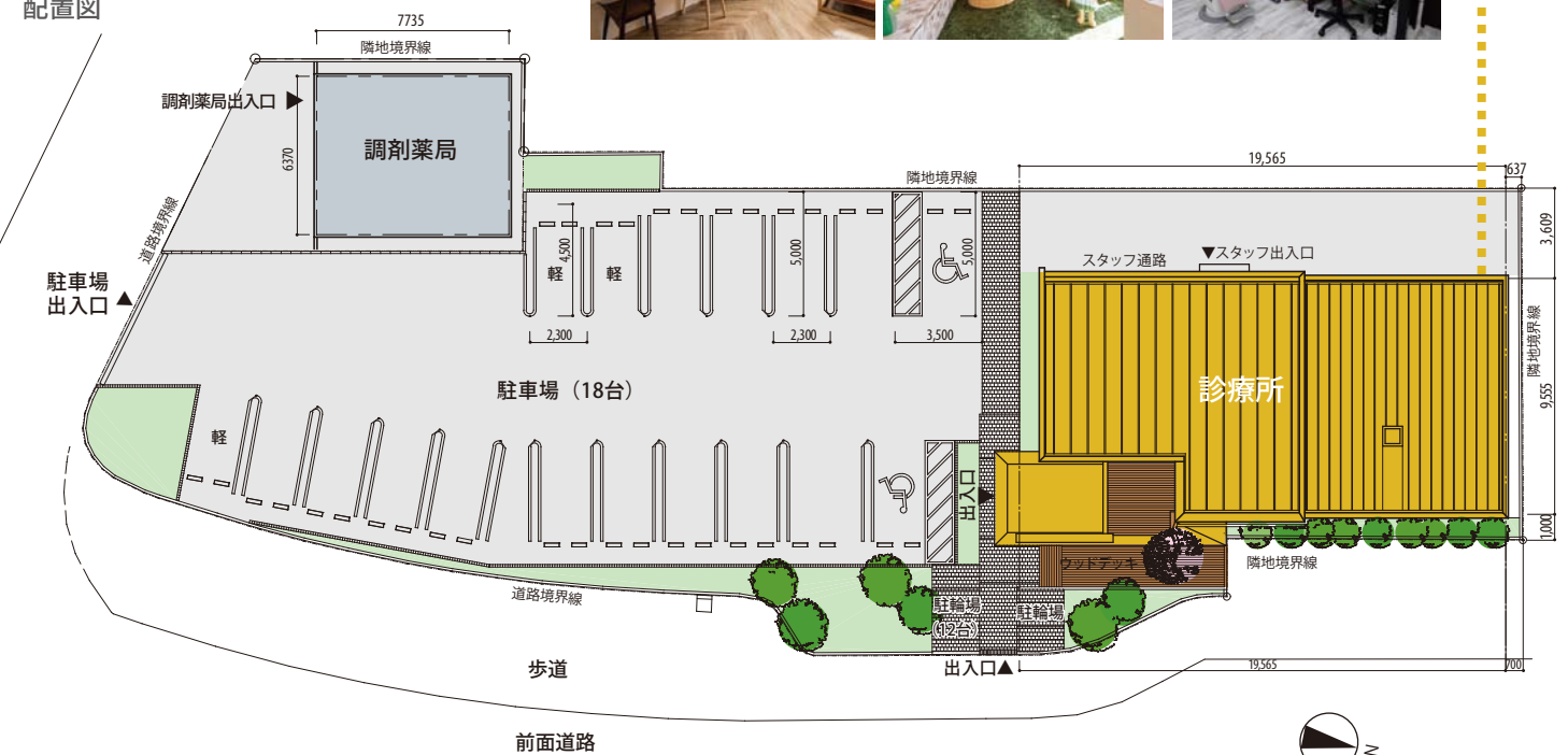
配置図
